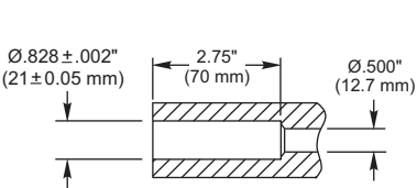
Section A-A (16X)
