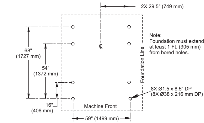
VF-7 Anchor Pattern
