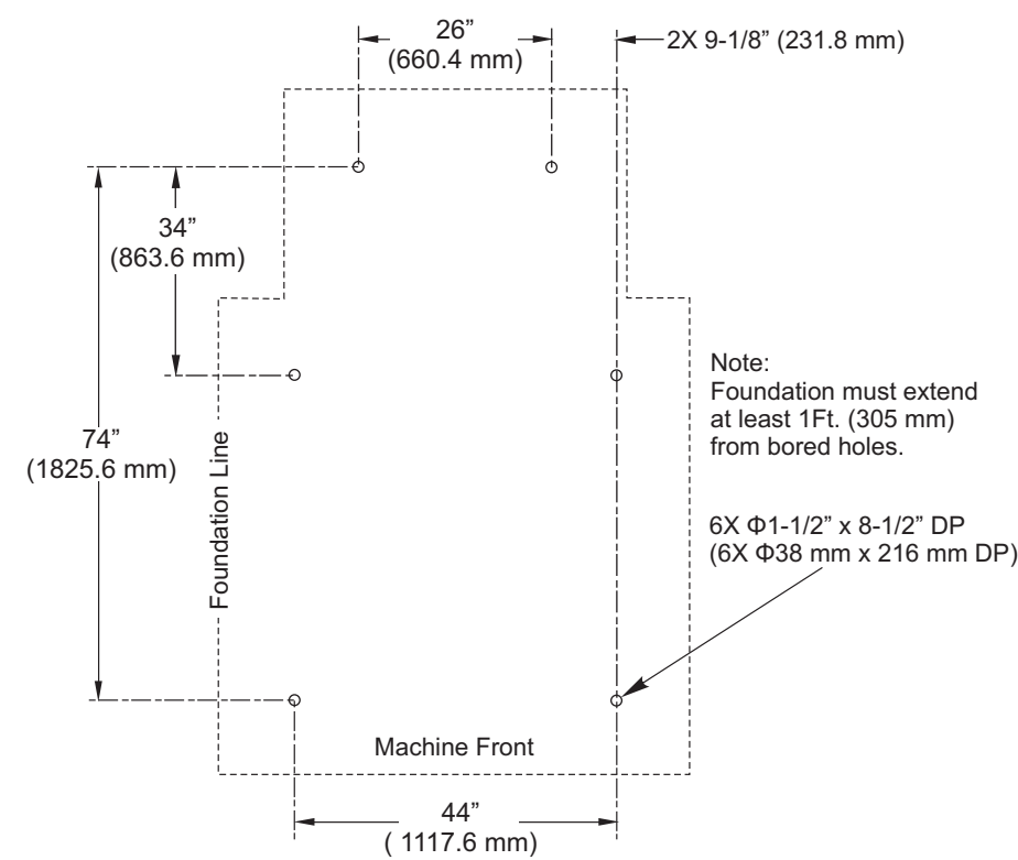
VF-3YT50 Anchor Pattern
